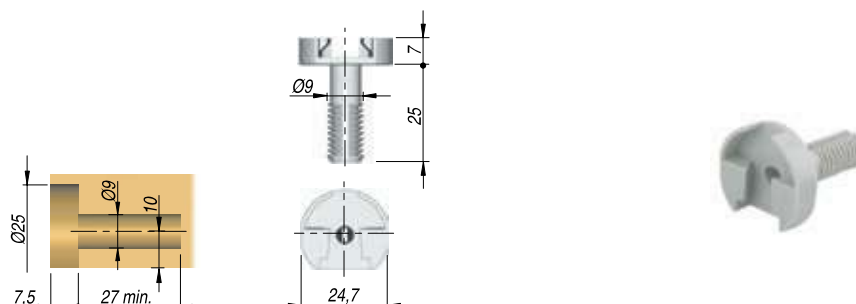
Tris 25mm - suporte de plástico para MDF
