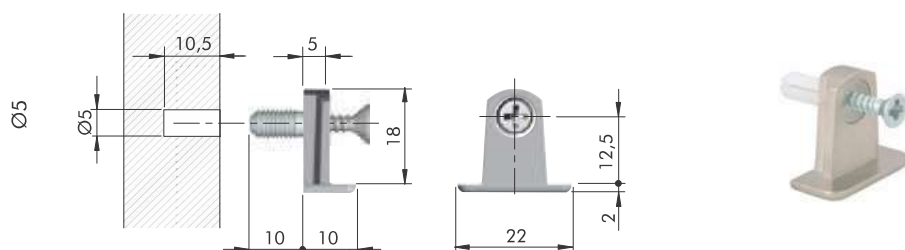
Tris 25mm - suporte metálico com bucha para MDF
